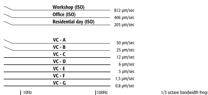
Graphique 2 : Critères vibratoires, VC
