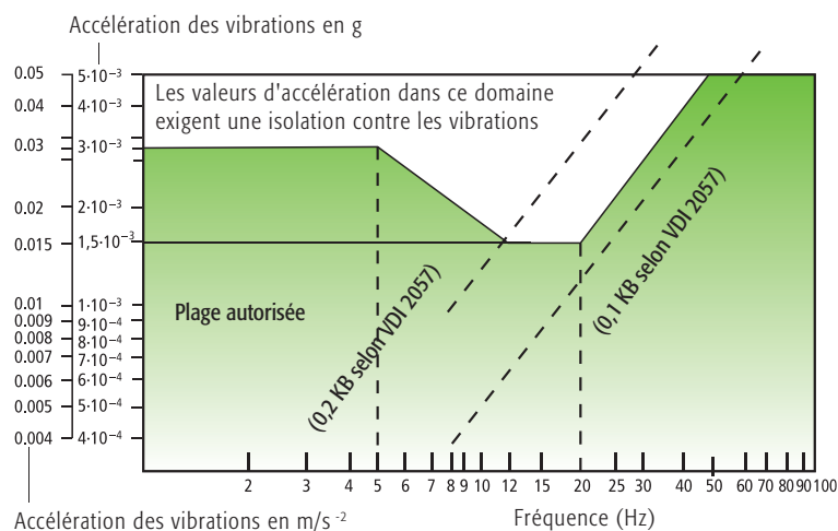
Graphique 1 : Exemple de courbe limite CMM
