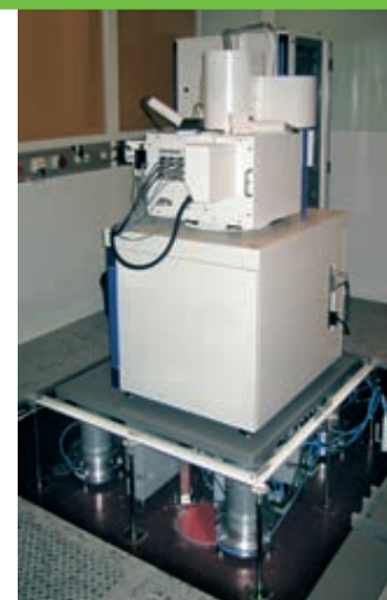
Exemple d'application : plateforme active pour microscopes électroniques
