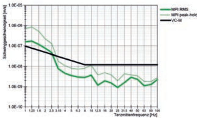
Résultat de la mesure des vibrations sur un bloc de fondations isolé avec des isolateurs pneumatiques à membranes Bilz.
