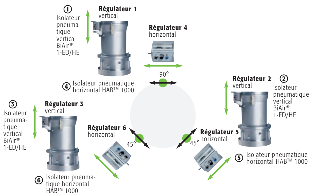
Exemple d'application : plateforme active pour microscopes électroniques
